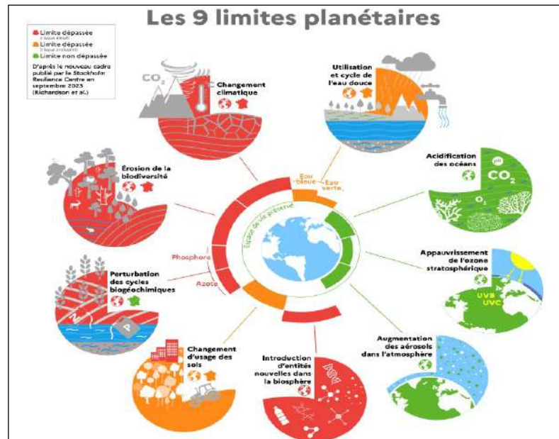
Figure n°8 : Les six limites planétaires franchies en septembre 2023
